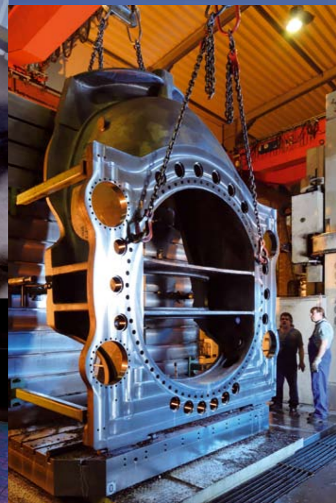
Grundrahmen für Windkraftanlage 7,6 t
