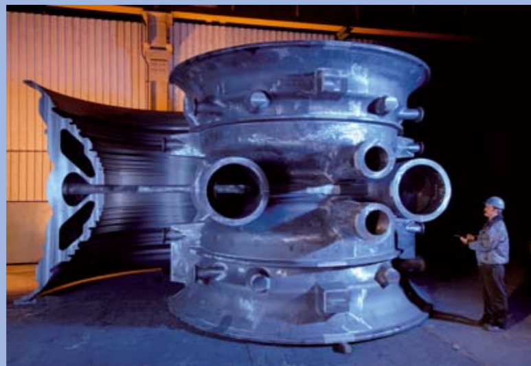
Endkontrolle von Dampfturbinenteilen Final inspection of steam turbine casing
