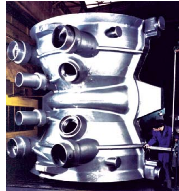
Dampfturbinen-Innengehäuse für die USA Steam Turbine Inner Casing for the USA
