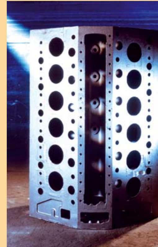
Zylinderkurbelgehäuse 2,9 t Crank Case 2,9 t
