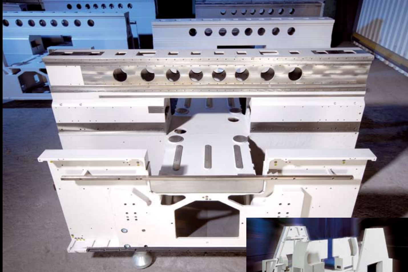
Maschinenständer 2,1 t Machine frame 2,1 t
